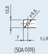
접속도체 가공도
