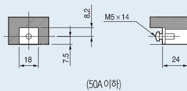
단자부 상세도
