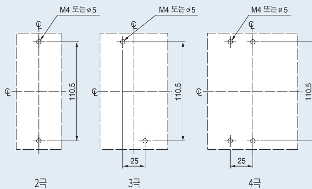
패널설치치수
