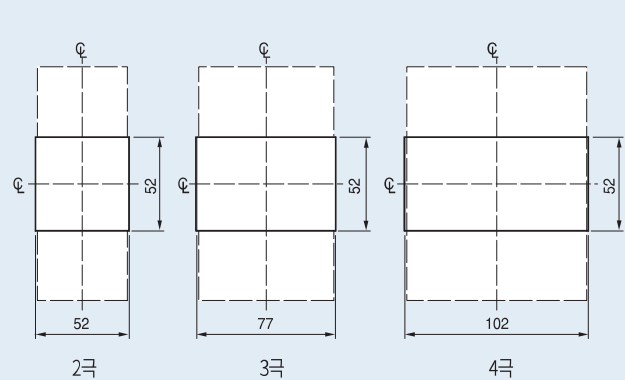
패널커버절단치수
