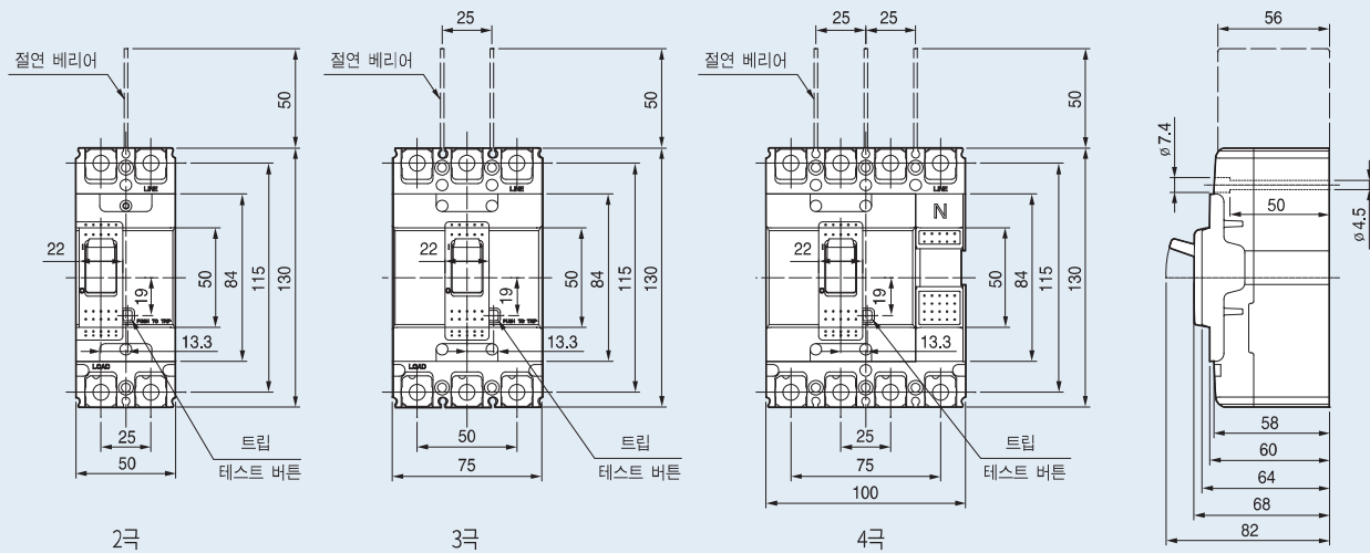
단자부 상세도
